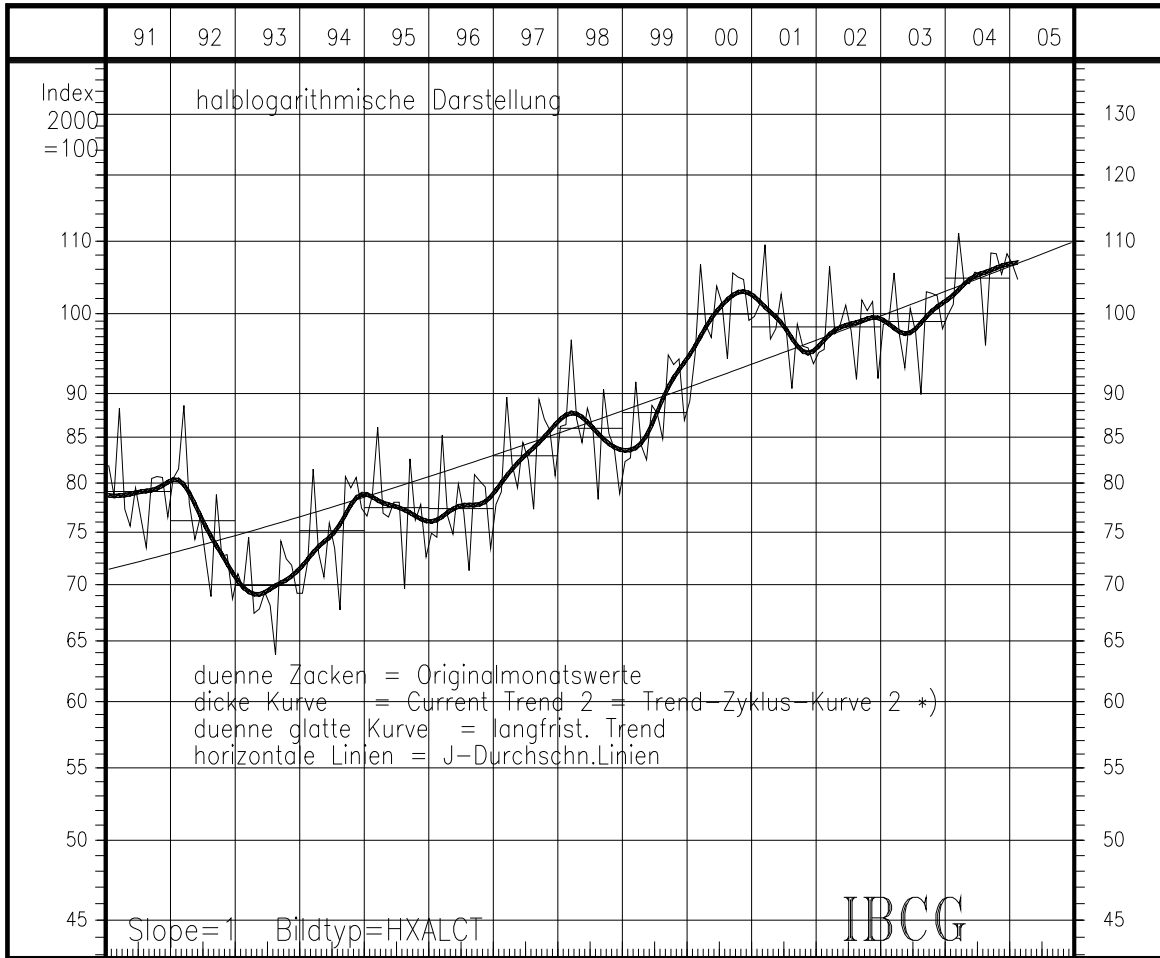
UXA001 D-Ges: Verarb. Gewerbe (DB-DN): Auftr.Eingang insges. Werte (at ber.) 2000=100 Orig.Werte
