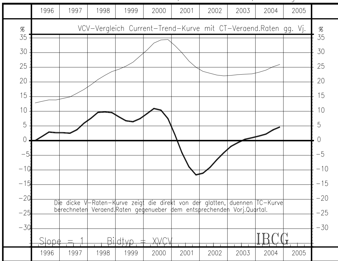
QX88Q1 D-Ges: VGR: Ausr.Investitionen, real Mrd Euro, SVR-Prognose ab 2003-3
